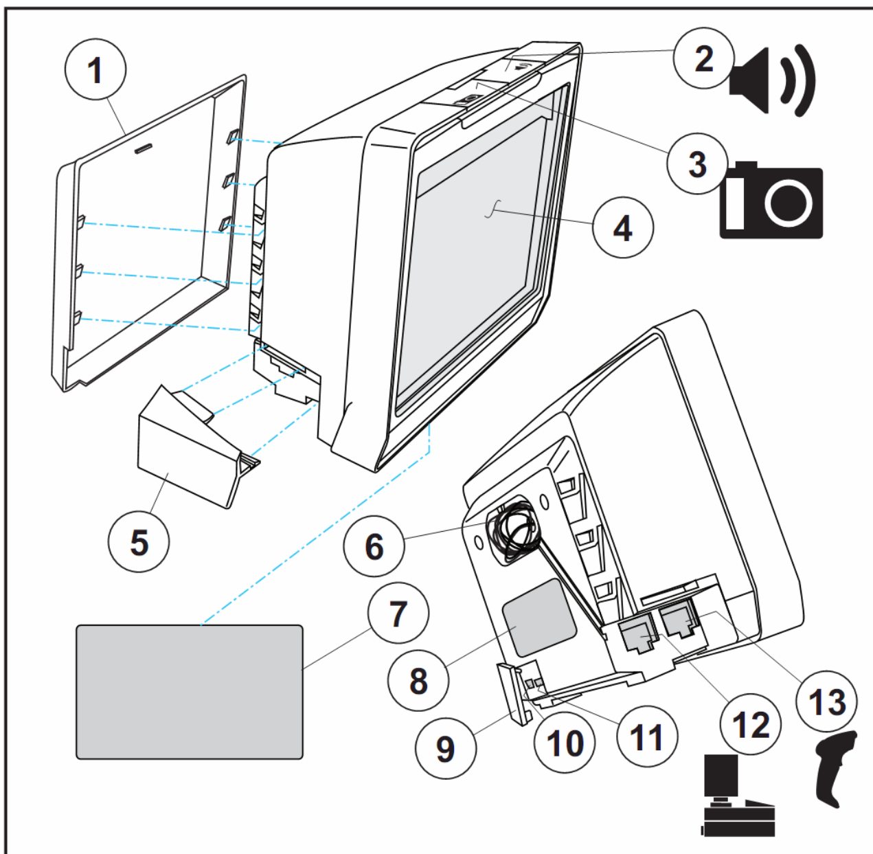
Rysunek 1. Budowa czytnika
